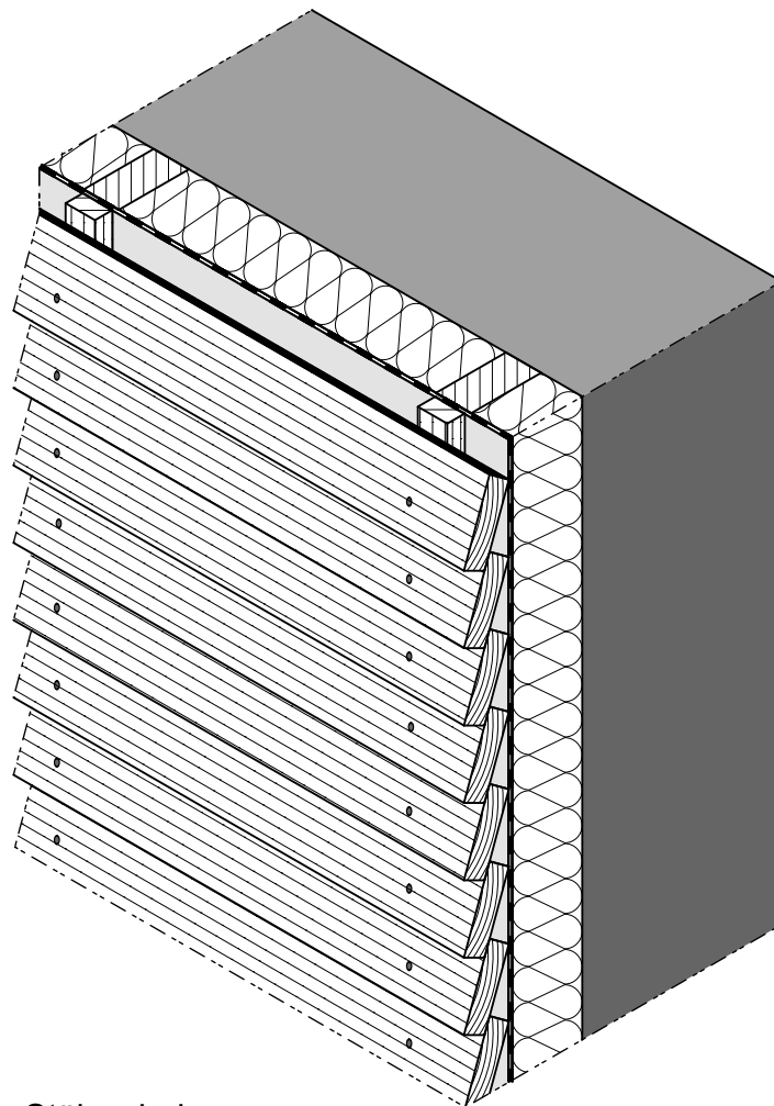
Stülpchalung
