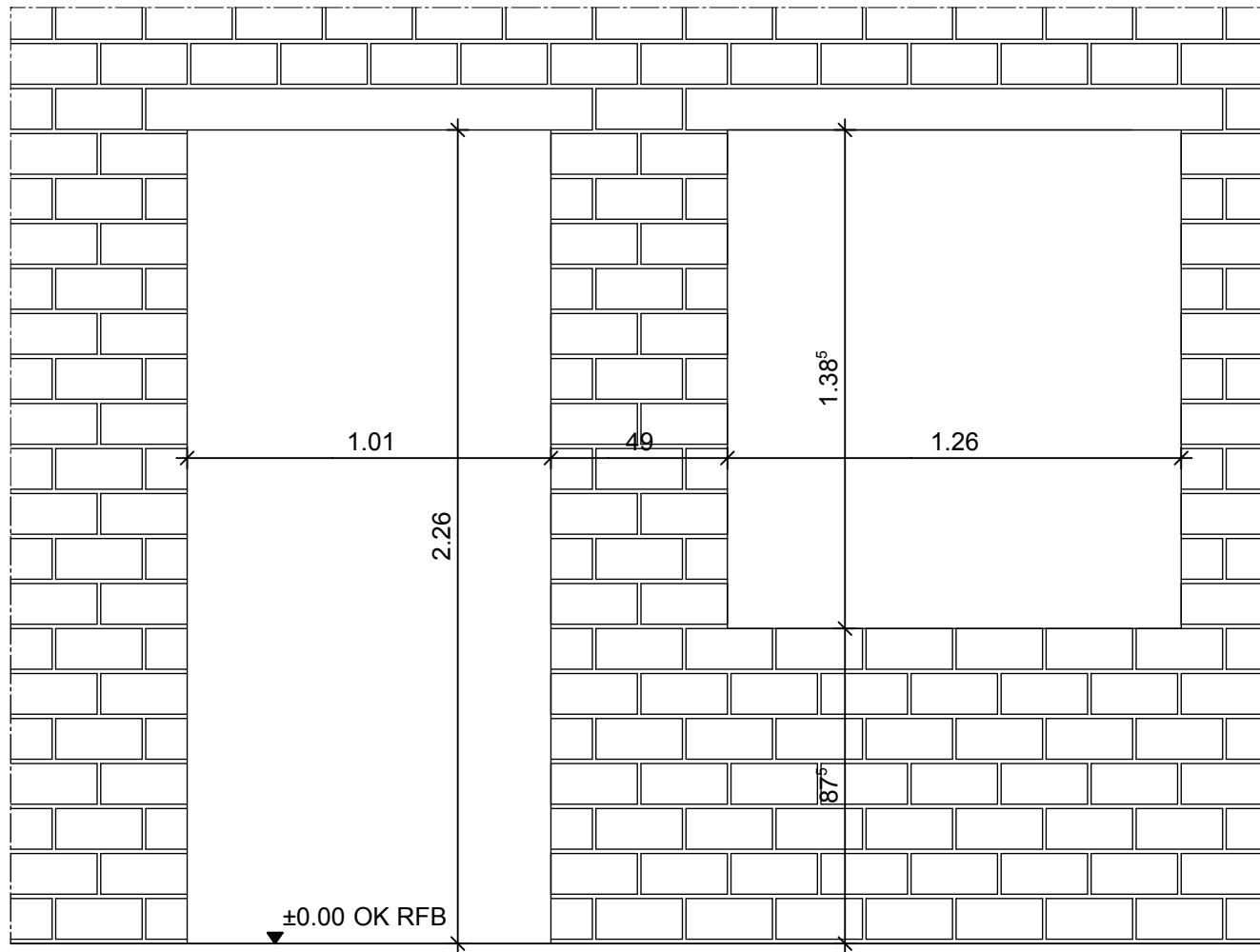
Beispiel für Rohbauöffnungsmaße
