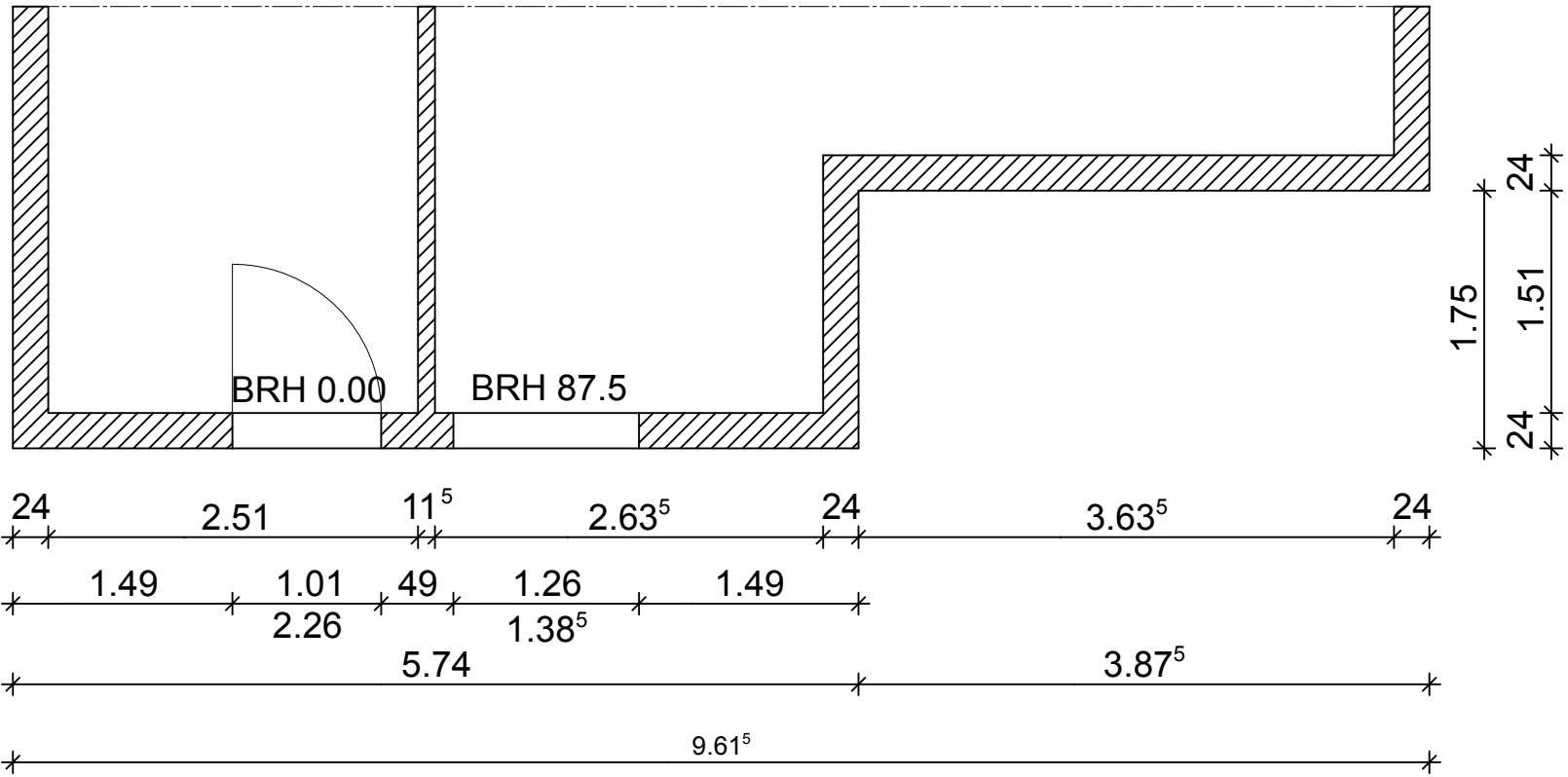
Beispiel für Mauerwerksmaße im Grundriss
