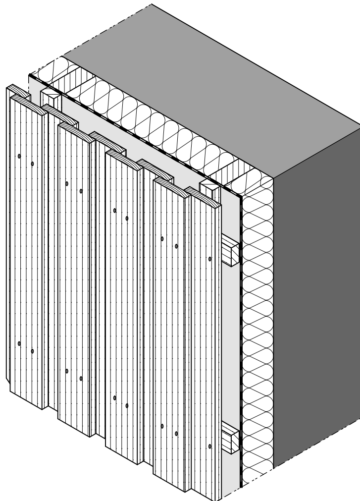
Deckelschalung
